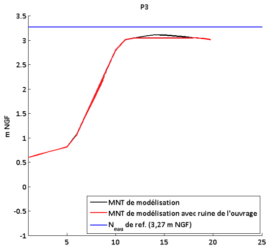
Comparaison des MNT avec et sans ruine pour les profils P3 et P4
