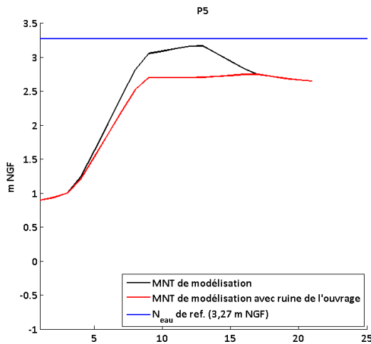
Comparaison des MNT avec et sans ruine pour les profils P5 et P6
