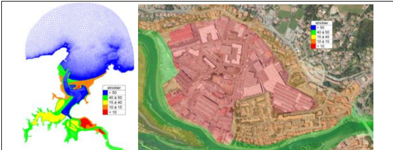
Figure 37 - Carte de répartition des coefficients de Strickler ( m^{1/3} s^{-1} ) exprimant la rugosité du sol.
