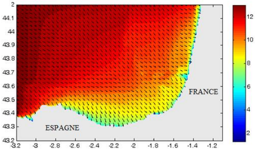
Figure 34 : Exemple de résultats de simulation réalisée avec le modèle SWAN sur le modèle de grande entreprise. Hauteur significative des vagues (m).
