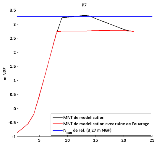
Comparaison des MNT avec et sans ruine pour les profils P7 et P8
