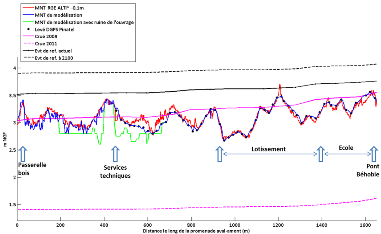
Figure 46 : Présentation des niveaux d'eau simulés le long de la promenade des Joncaux comparativement aux niveaux des crues passées (2009 et 2111).
