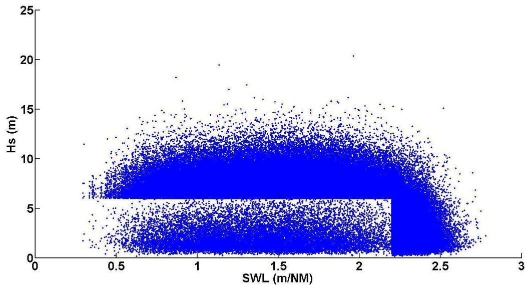
Figure 31 : Couples (H_s, SWL) initiaux superposés aux données simulées par JOIN-SEA (10 000 ans).
