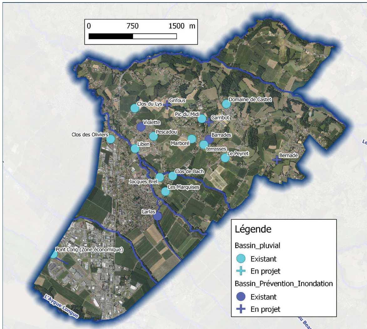
Fig. 13. Localisation des ouvrages de rétention
