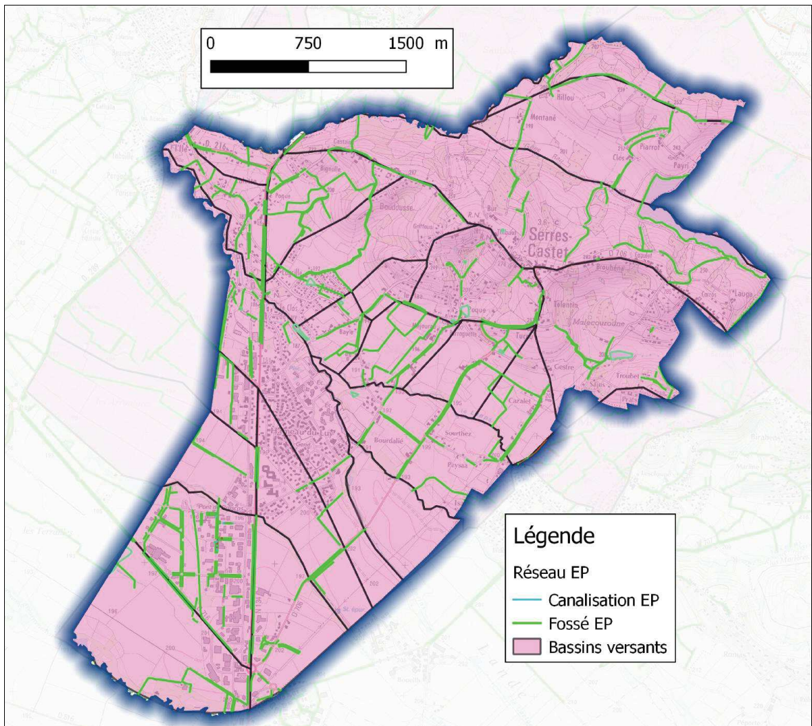
Fig. 8. Bassins versants de la commune
