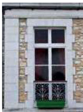
Encadrement pierre de taille, piédroits harpé. Lasseube.
